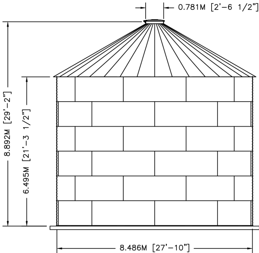
ELEVATION
